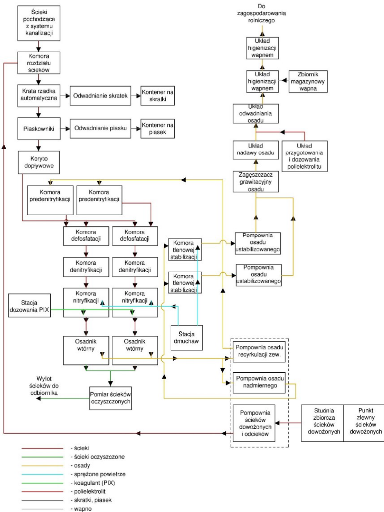
Rysunek 1_ Schemat blokowy funkcjonujących obiektów oczyszczalni ścieków w Krasnymstawie _ Stan aktualny
